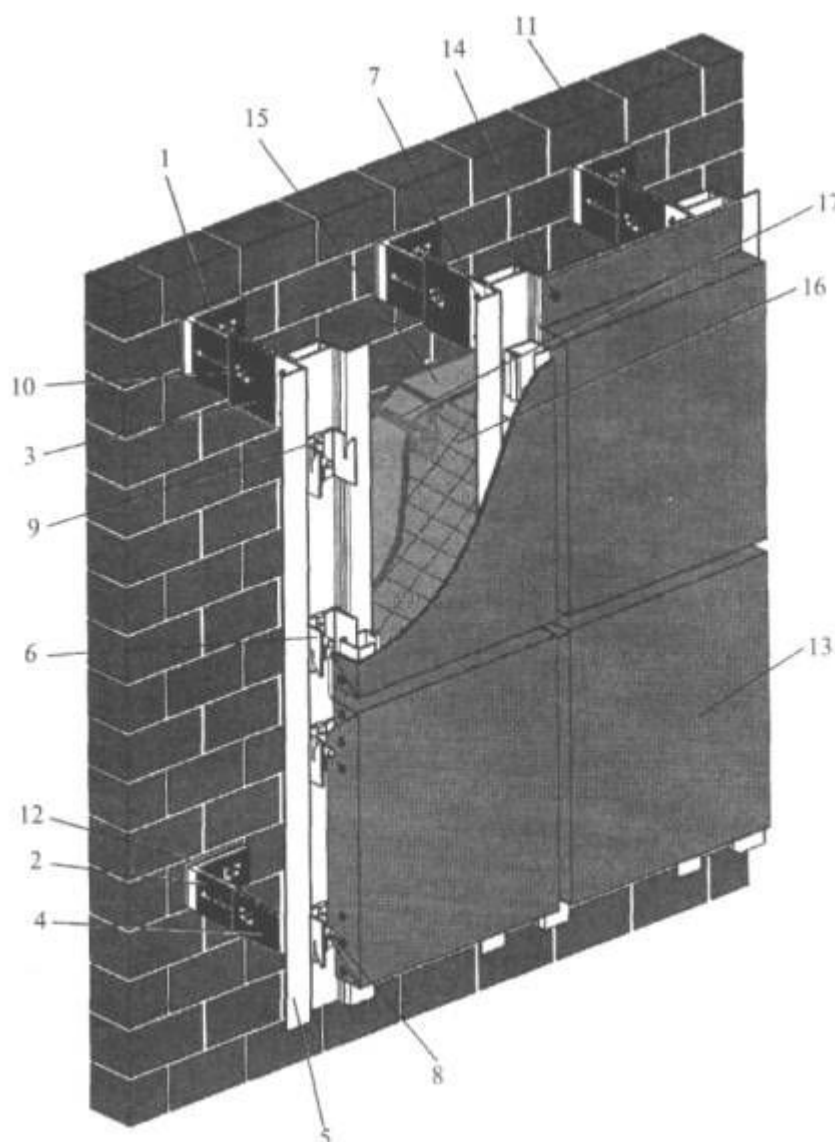
Рис. 1. Фрагмент фасада системы FS-300
