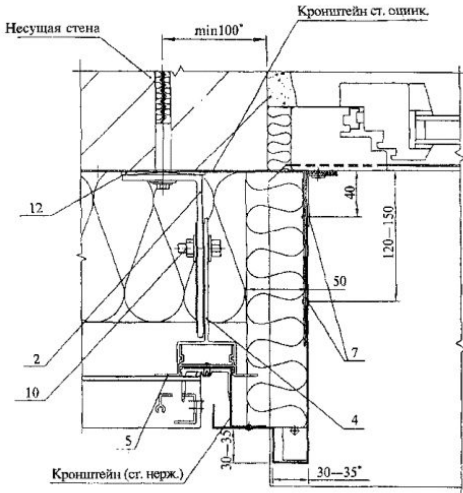
Рис. 11. Примыкание к оконному проему (сбоку)
