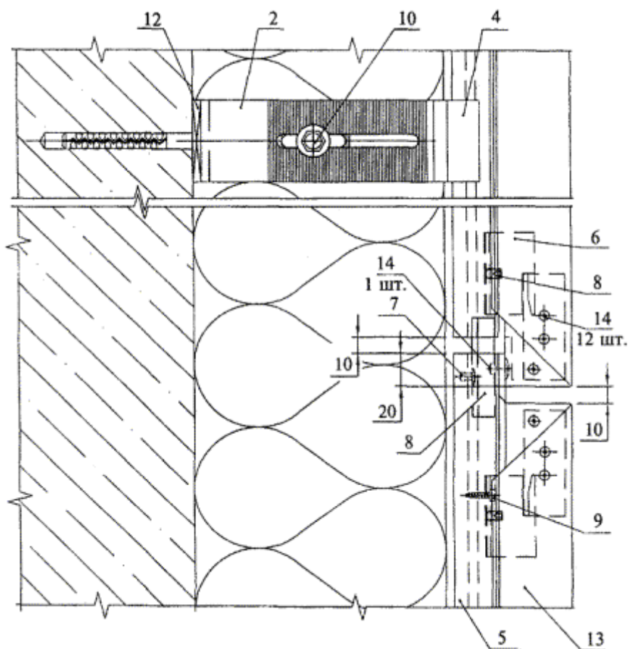
Рис. 7. Установка облицовочных панелей на стыке несущих профилей
