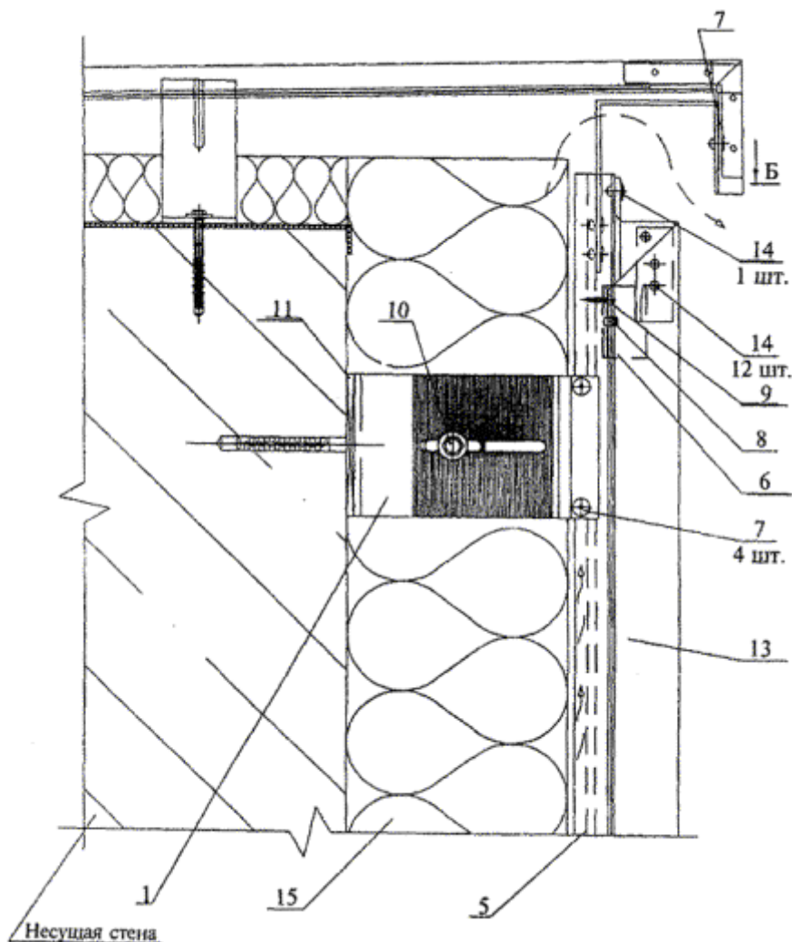
Рис. 13. Узел примыкания к парапету
