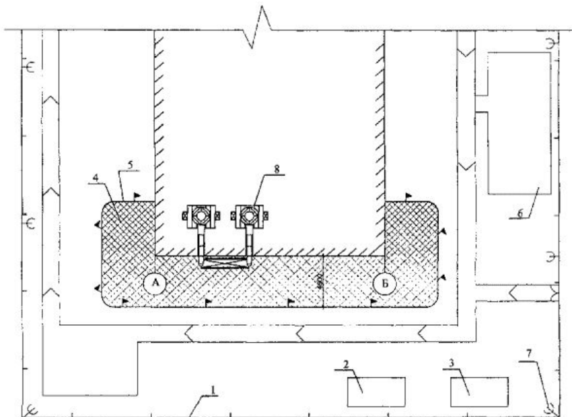
Рис. 2. Схема организации строительной площадки
