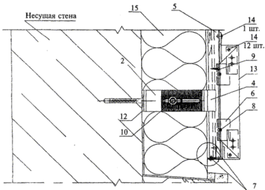
Рис. 5. Узел примыкания к цоколю Вертикальный разрез
