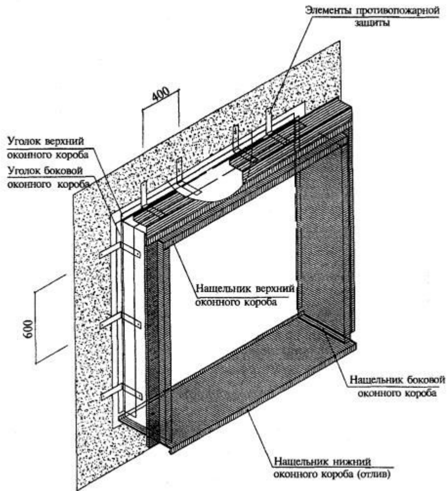
Рис. 9. Общий вид оконного обрамления
