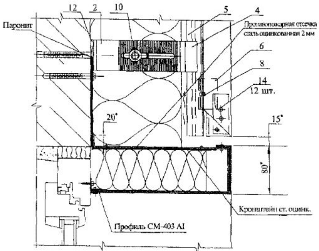
Рис. 11. Примыкание к оконному проему (сбоку)
