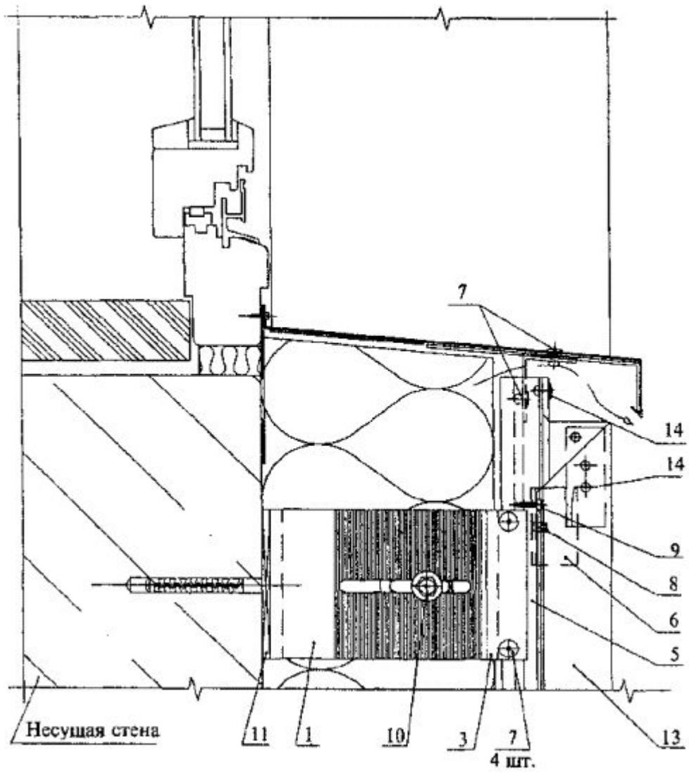
Рис. 10. Примыкание к оконному проему (нижнее) Горизонтальный разрез
