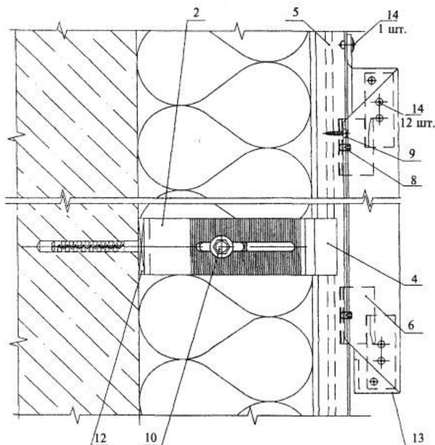
Рис. 5. Узел примыкания к цоколю Вертикальный разрез
