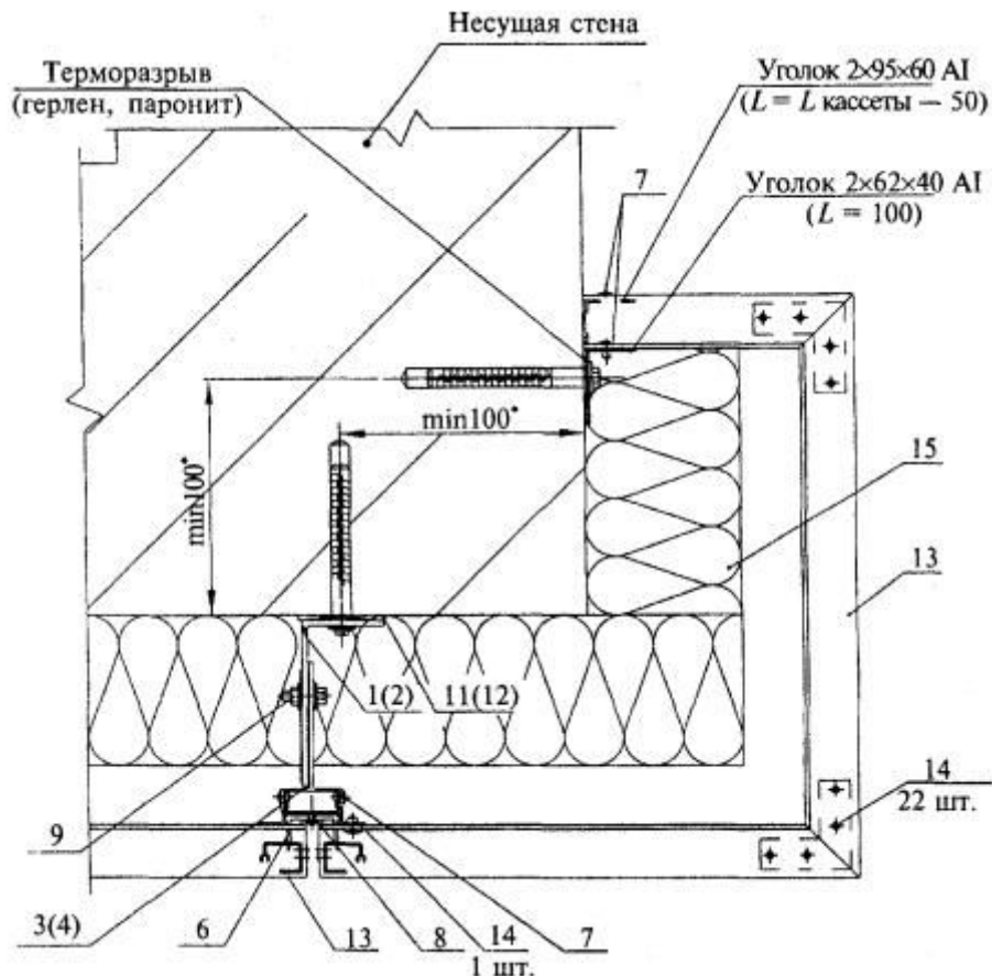
Рис. 8. Узел крепления облицовочных панелей на наружном углу здания
